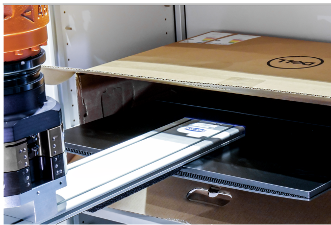
エアグリッパー FEL ハンドリングスクリーン
