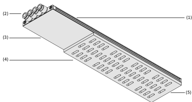
システムデザイン 薄型真空グリッパー FEL
